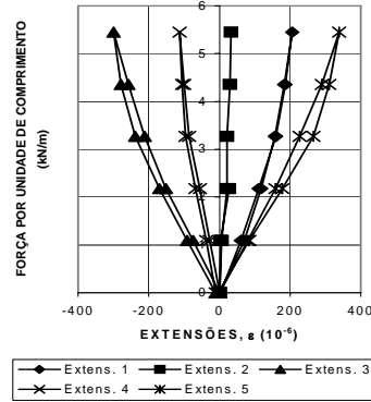
Figura 6 – Fase de exploração (Lâmina 1) (Carga ao centro, em 55 mm).
