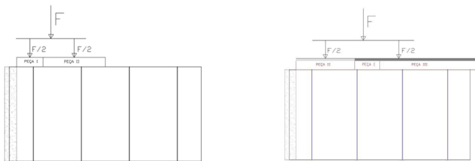
Figura 4 – Representação esquemática da carga diferenciada em 185 mm (a) e da carga diferenciada em 385 mm (b).
