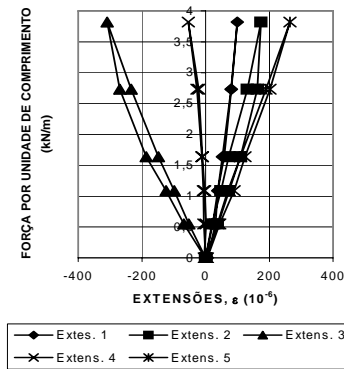
Figura 5 – Fase de construção (Lâmina 3) (Carga ao centro, em 55 mm).
