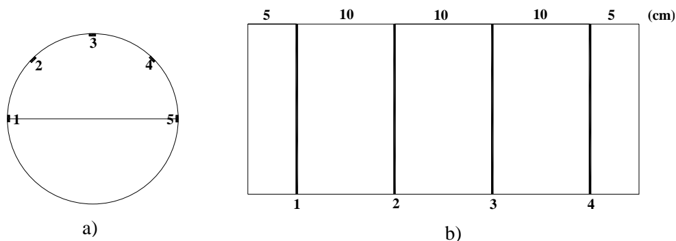
Figura 1 – Representação esquemática da localização dos extensómetros na secção do tubo (a) e localização das lâminas ao longo do comprimento do referido tubo(b).
